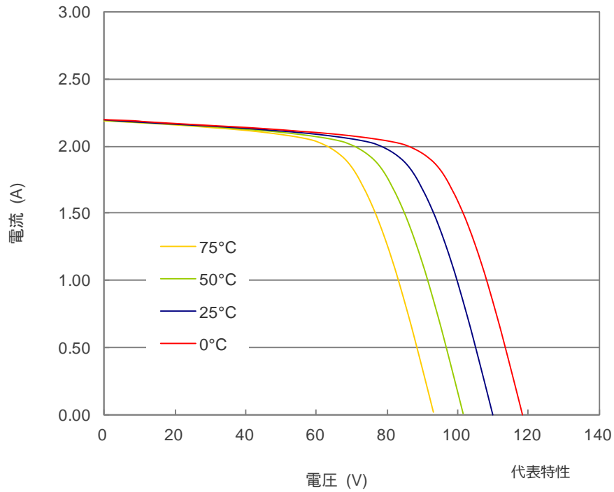
モジュール温度別 I-V特性 型式 : SF160-S 測定条件 : AM 1.5 1000W/m 2
